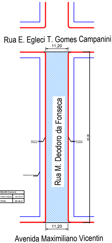
PLANTA DO TRECHO DE RECAPE Escala:.....1/400
