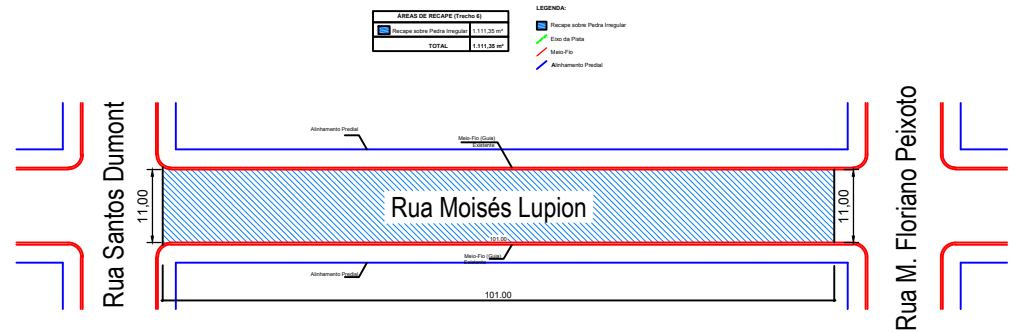
PLANTA DO TRECHO DE RECAPE Escala:.....1/400
