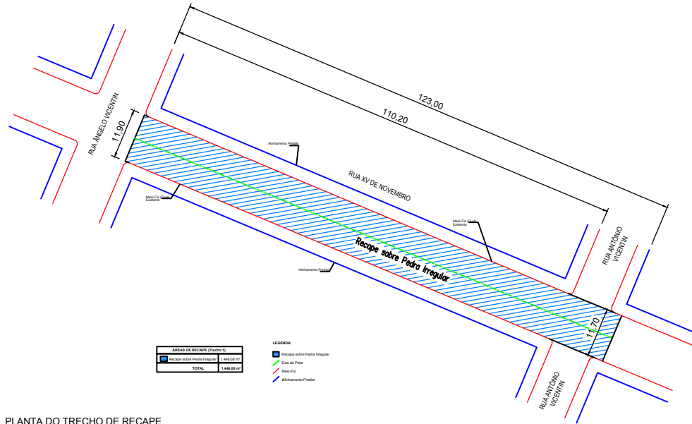
PLANTA DO TRECHO DE RECAPE Escala:.....1/400
