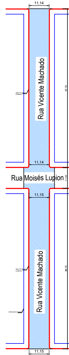
PLANTA DO TRECHO DE RECAPE Escala:.....1/400
