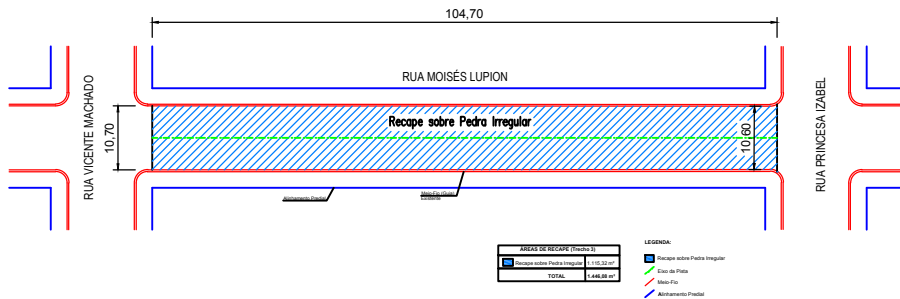
PLANTA DO TRECHO DE RECAPE Escala:.....1/400
