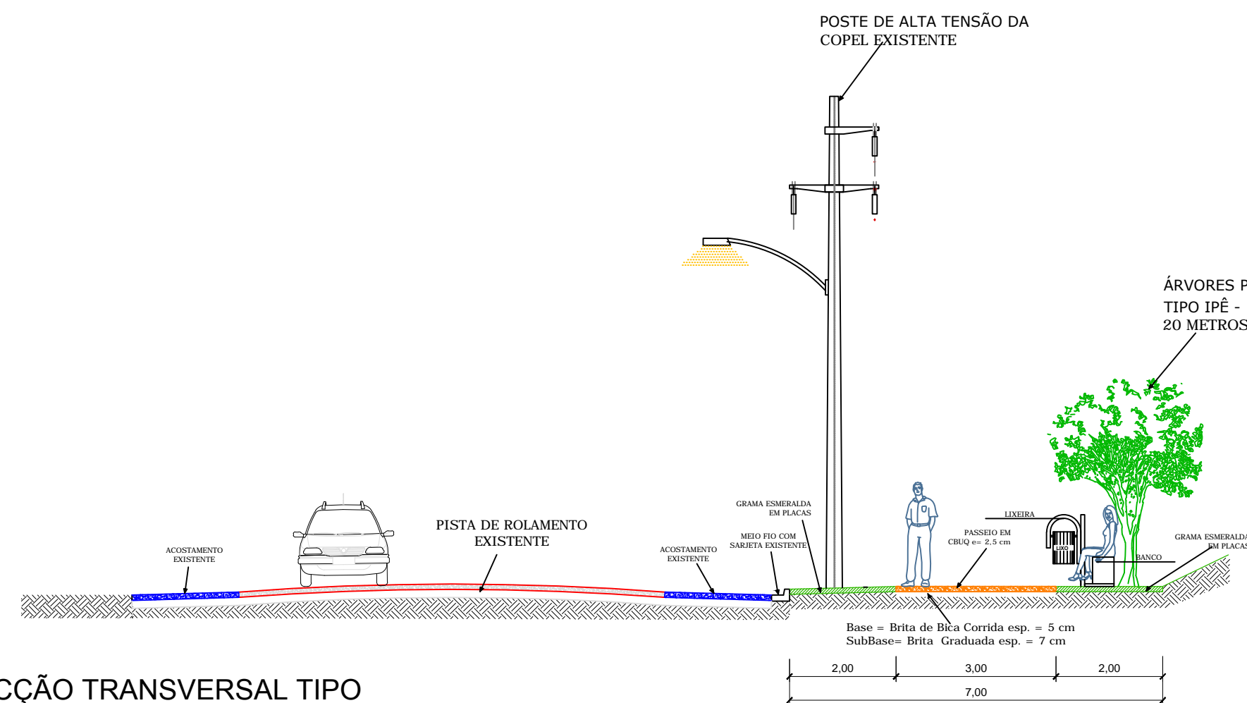
SEÇÃO TRANSVERSAL TIPO
