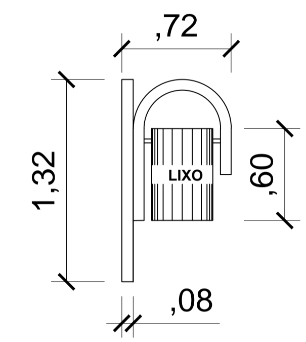
Detalhe Lixeira Escala 1:25
