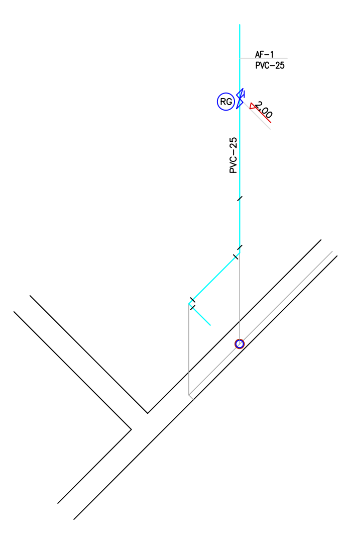
DETALHE ISOMÉTRICO - LAVA CAR ESCALA:.....1:25
