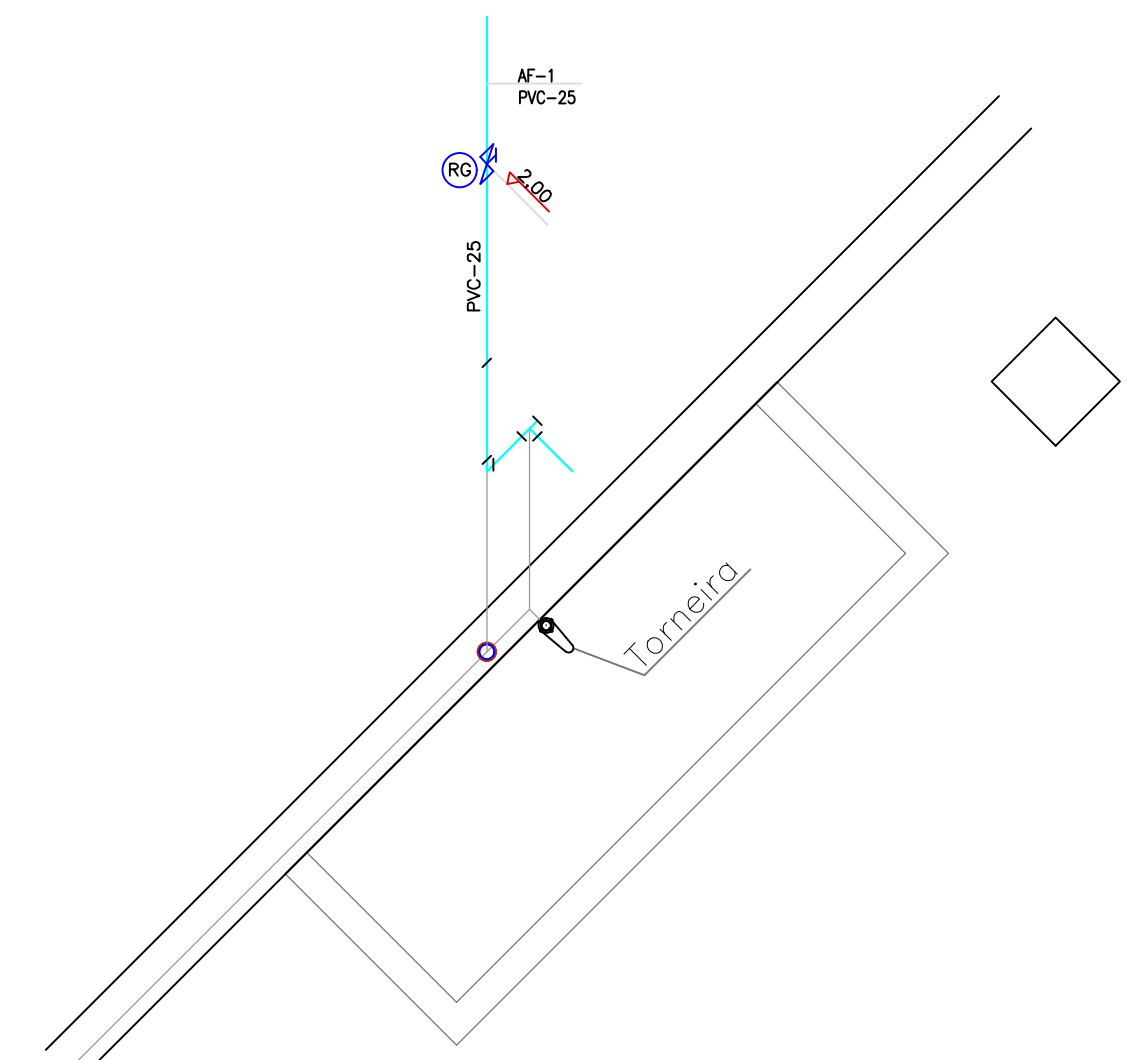
DETALHE ISOMÉTRICO - LAVA PEÇAS ESCALA:.....1:25
