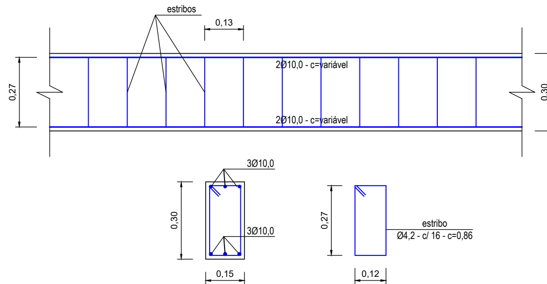
DET. ARMAÇÃO VIGA CINTA escala 1:15
