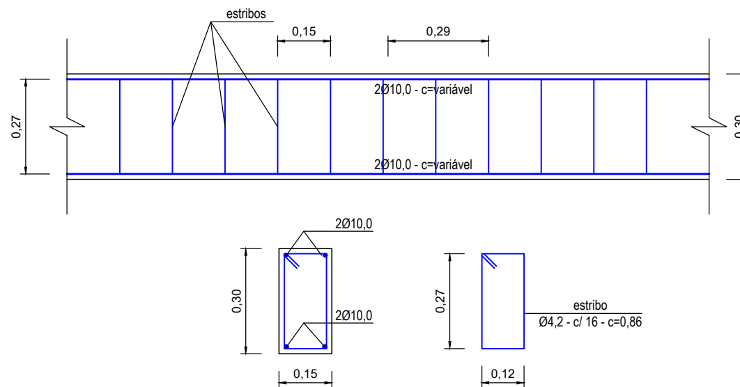
DET. ARMAÇÃO VIGA BALDRAME escala 1:15
