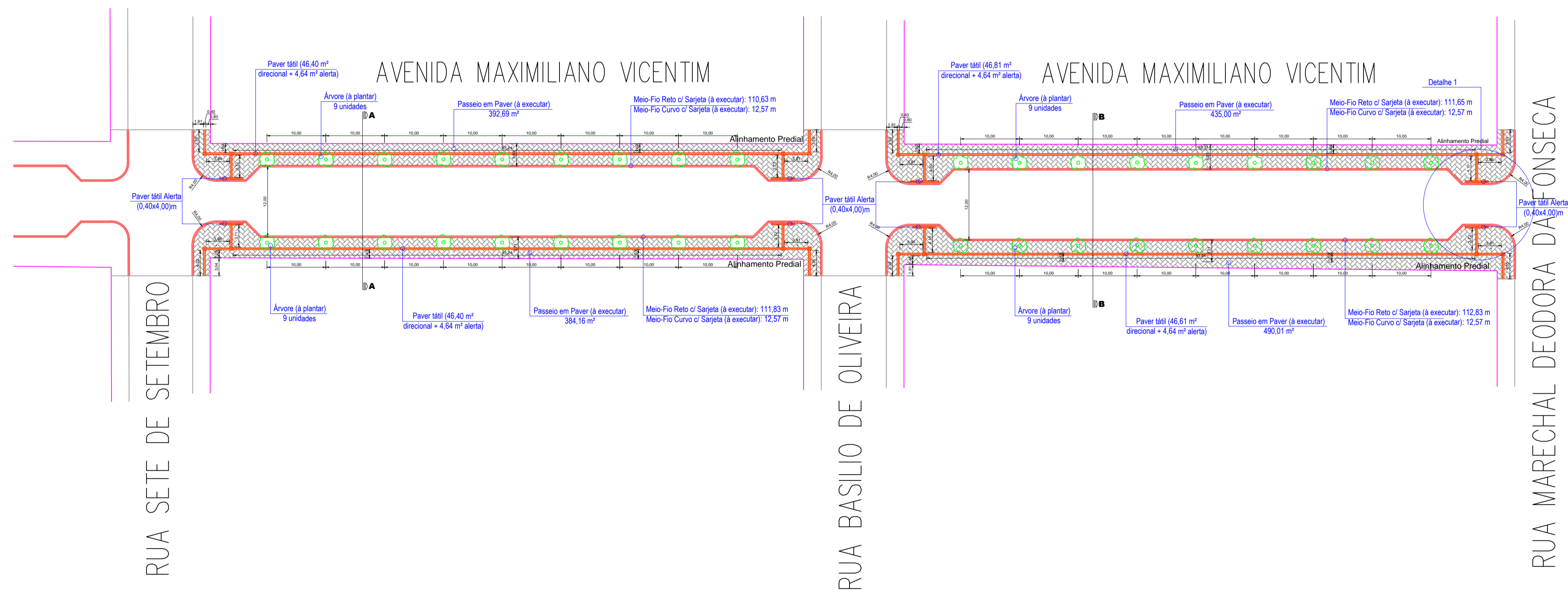
PLANTA DOS EQUIPAMENTOS URBANOS Escala:.....1:500
