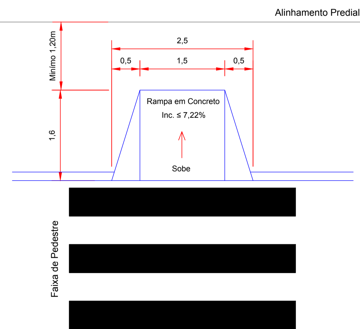
Rampa de Acessibilidade (detalhe) - TIPO 1 Esc.: 1:25
