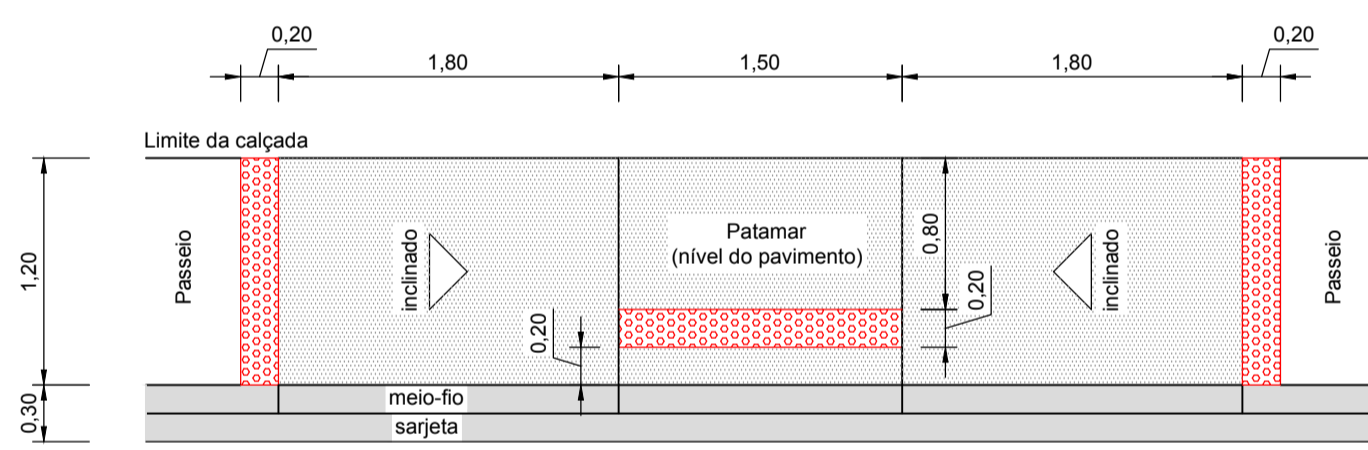
Rampa de Acessibilidade (detalhe) - TIPO 2 Esc.: 1:25
