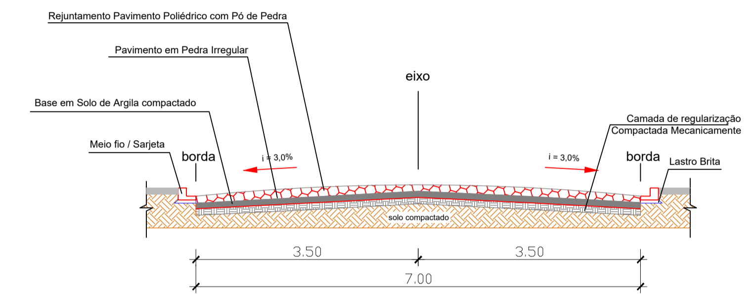
Secção Transversal (Corte AA) escala 1:50
