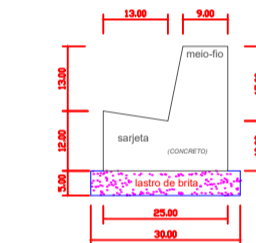
Secção Transversal Tipo escala 1:10
